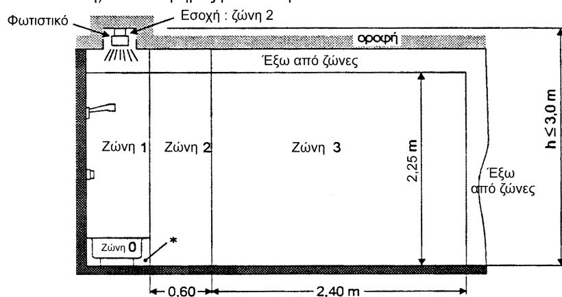
θ) Καταιονητήρας χωρίς λεκάνη + σταθερό χώρισμα
