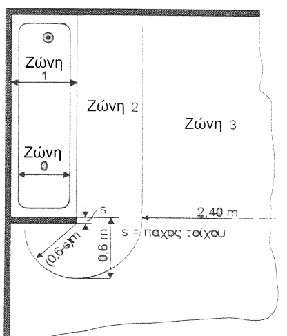
δ) Καταιονητήρας με λεκάνη + σταθερό χώρισμα
