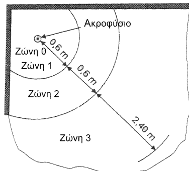
ε) Καταιονητήρας χωρίς λεκάνη. Σταθερό ακροφύσιο
