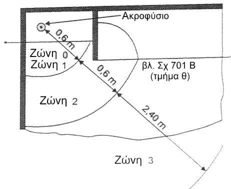
στ) Καταιονητήρας χωρίς λεκάνη + σταθερό χώρισμα. Σταθερό ακροφύσιο
