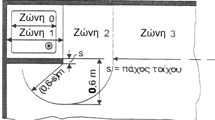
δ) Καταιονητήρας με λεκάνη + σταθερό χώρισμα
