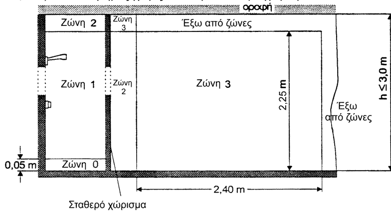
Σχ 701 Β. Διαστάσεις ζωνών (πλάγια όψη). Το σχέδιο δεν είναι υπό κλίμακα
